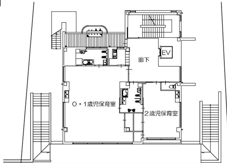
【2階平面図】
