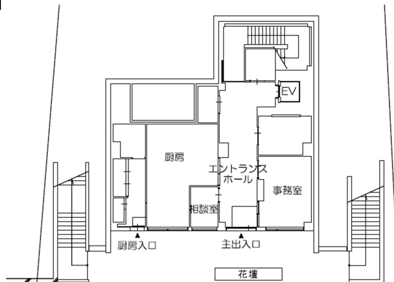
【1階平面図】
