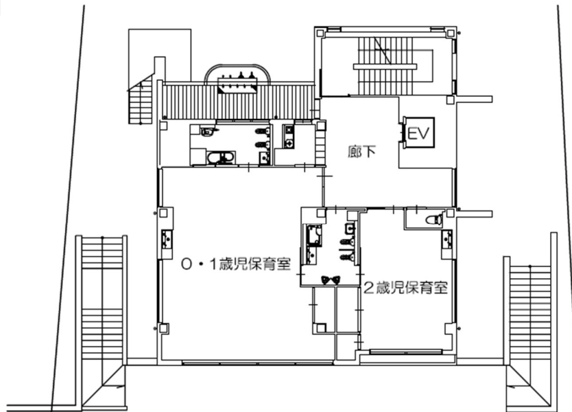
【2階平面図】
