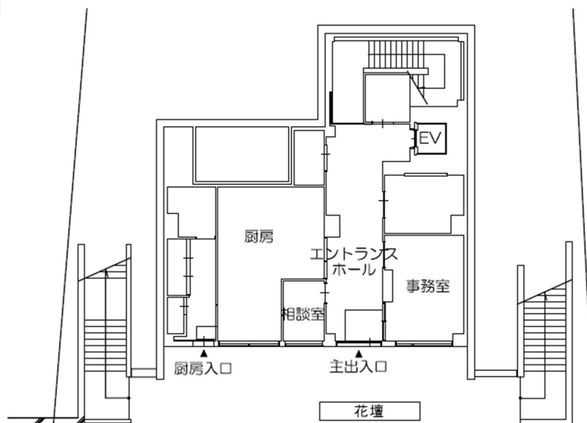
【1階平面図】
